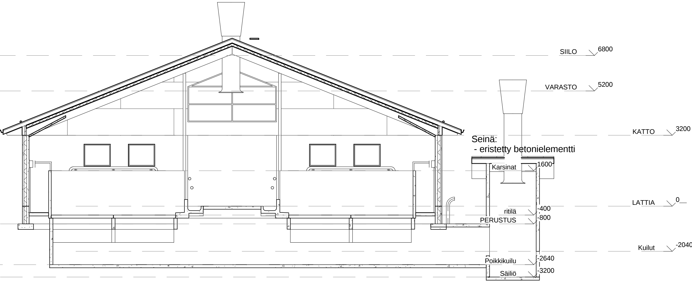
Poikkileikkaus
